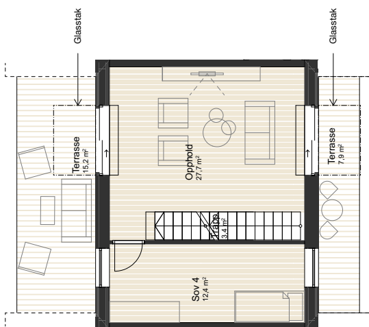
3. etasje
